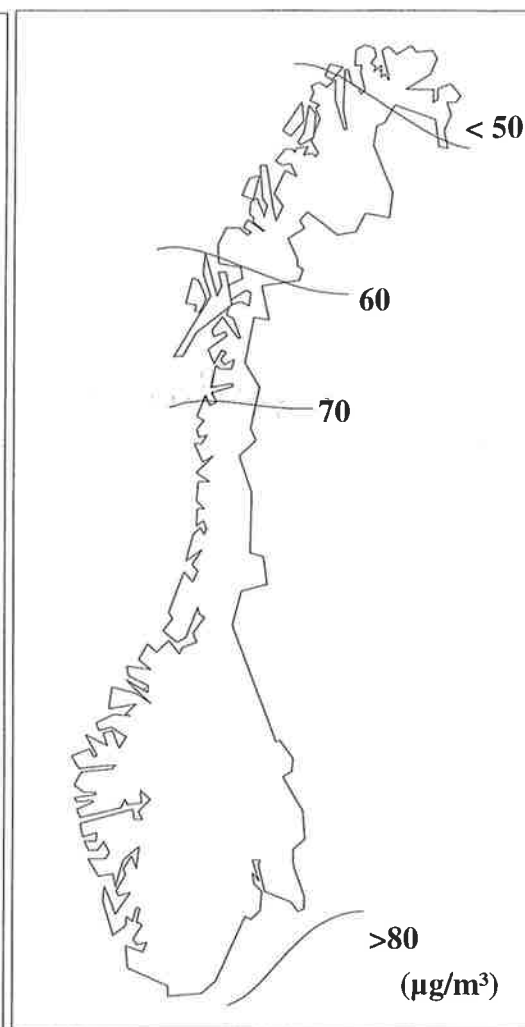
Figur 4.3: Midlere 7 h-konsentrasjon av ozon ( \mu\text{g}/\text{m}^3 ) kl. 09-16, april-september 1996.
