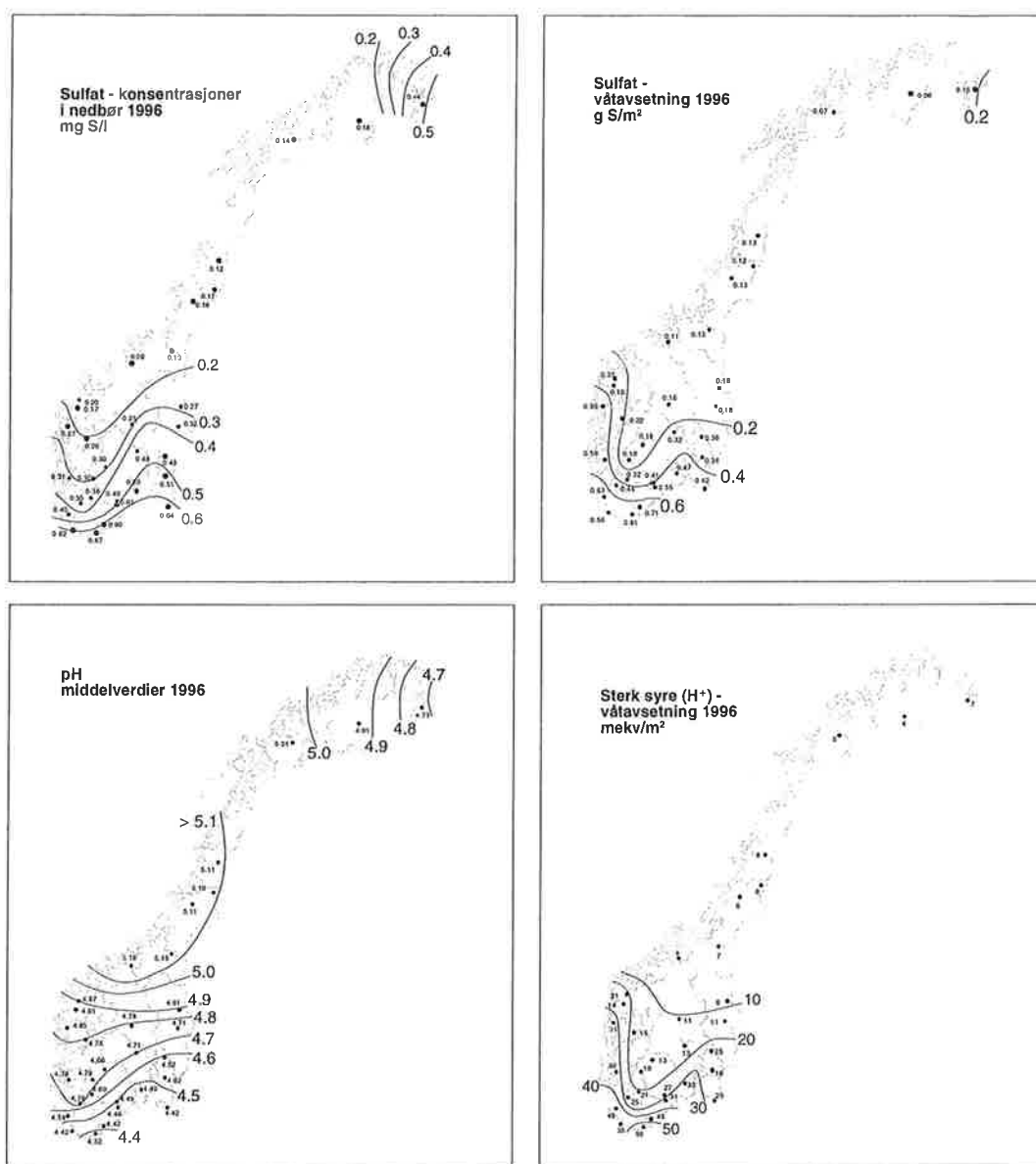
Figur 1.1: Middelkonsentrasjoner i nedbør og våtavsetning av sulfat (sjøsaltkorrigert) og sterk syre (pH) på norske bakgrunnsstasjoner i 1996.
