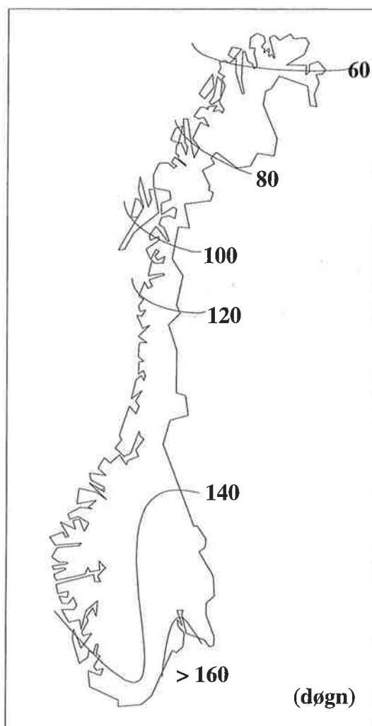
Figur 4.2: Antall døgn med 8 h-middelverdier av ozon over 60 \mu\text{g}/\text{m}^3 , april-september 1996.
