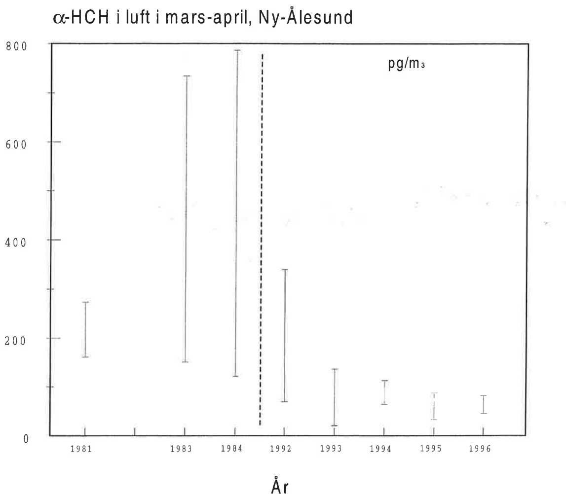
Figur 5.4: \alpha -HCH i luft i perioden mars-april i Ny-Ålesund.
