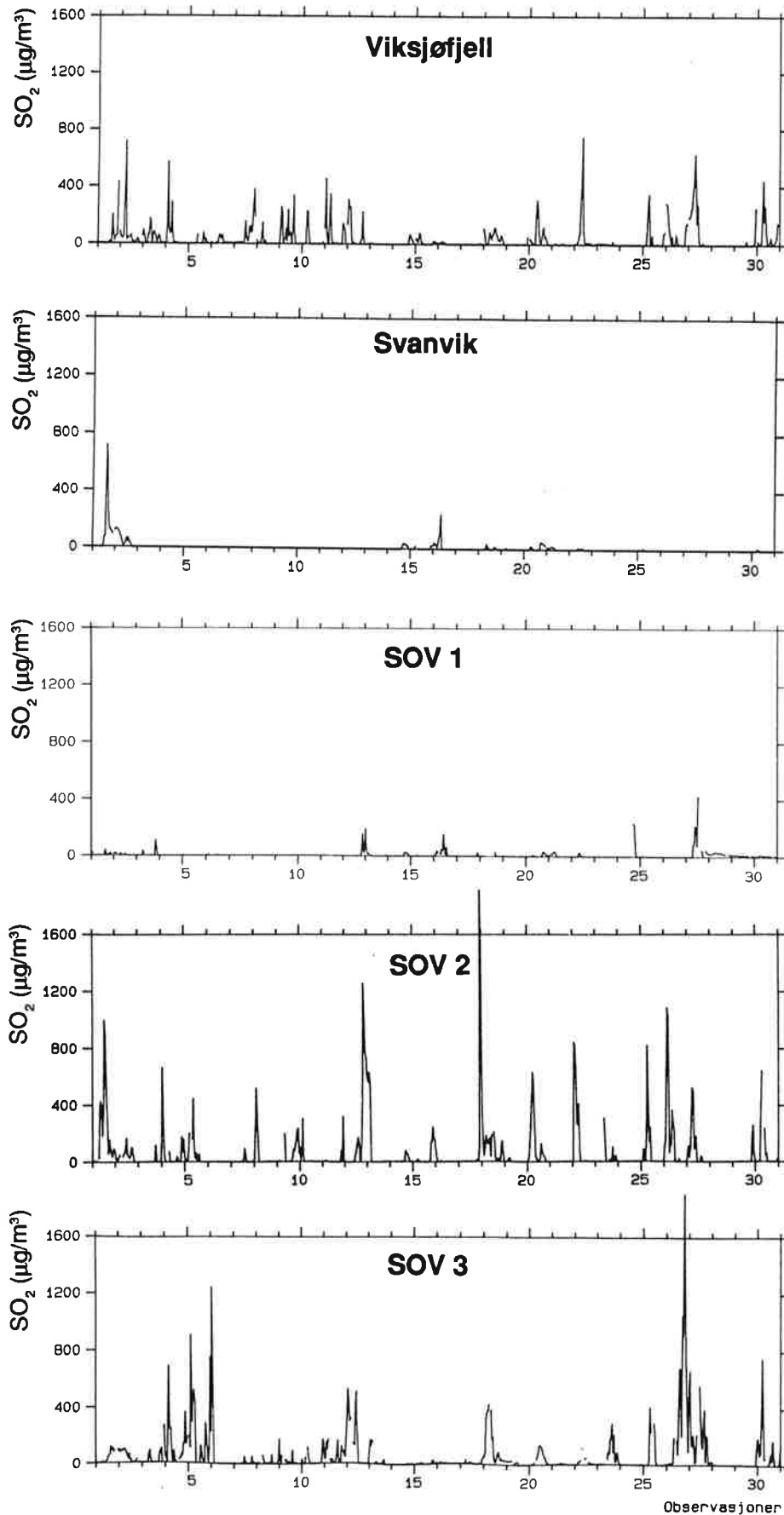
Figur 12: Timemiddelkonsentrasjoner av SO 2 i april 1991 på Viksjøfjell, Svanvik, SOV 1, SOV 2 og SOV 3 (µg/m 3 ).
