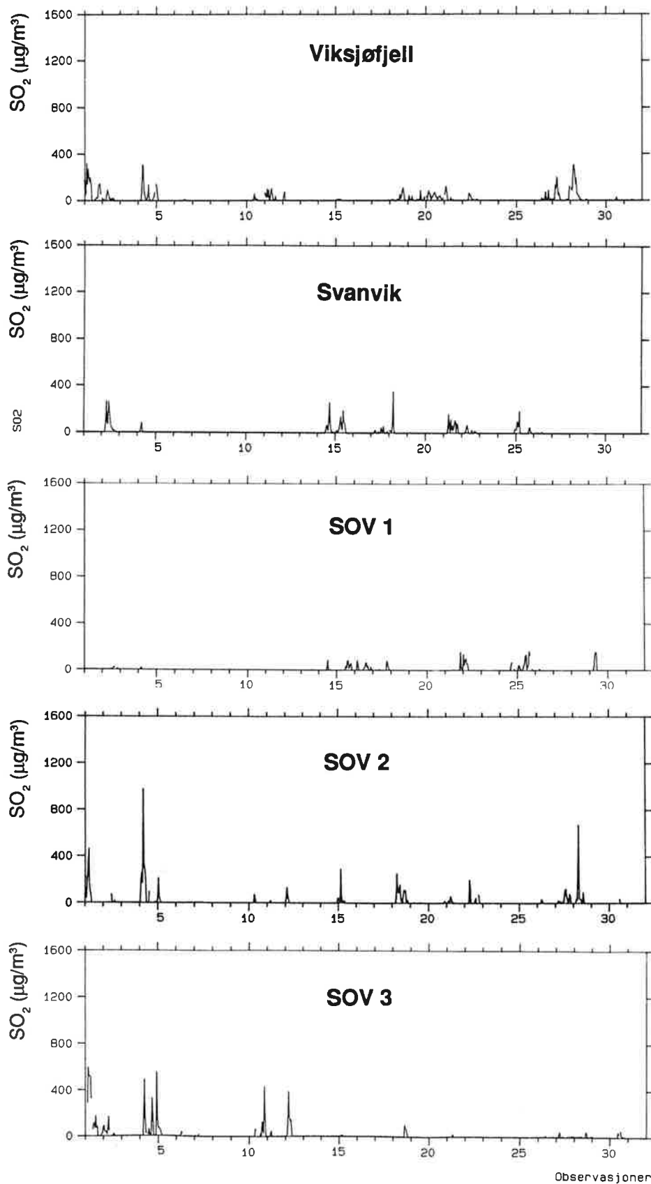
Figur 13: Timemiddelkonsentrasjoner av SO 2 i mai 1991 på Viksjøfjell, Svanvik, SOV 1, SOV 2 og SOV 3 (µg/m 3 ).
