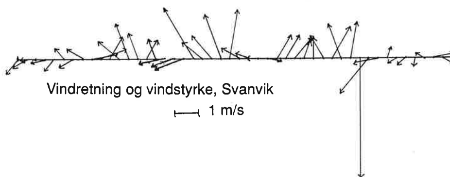
Figur 7: Timemiddelverdier av SO 2 , vindretning og vindstyrke 26.-27. juli 1991.
