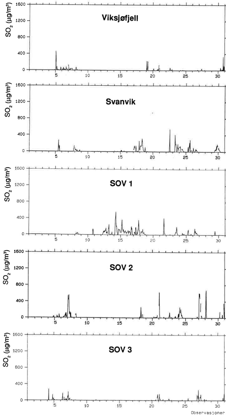
Figur 14: Timemiddelkonsentrasjoner av SO 2 i juni 1991 på Viksjøfjell, Svanvik, SOV 1, SOV 2 og SOV 3 (µg/m 3 ).
