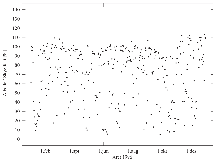
Figur 26: Effekter av skyer og bakkealbedo på UV-stråling ved jordens overflate i Oslo i 1996 i prosent av klarværsverdien med null bakkerefleksjon. Hvert punkt representerer middelerdien mellom 10:30 og 11:30 GMT for en bestemt dag. Den horisontale linjen representerer klarvær og barmark. Verdier over denne linjen betyr at skyer og/eller bakkealbedo øker UV-nivået sammenlignet med klarvær og bar bakke.
