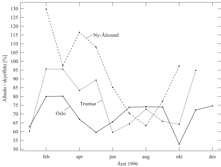
Figur 25: Albedo/skyeffekter for hver måned i 1996 målt med GUV-instrumentene i Oslo, Tromsø og Ny-Ålesund. Hvert punkt viser månedsverdien av UV-dosen i prosent av klarværsverdien med null bakkerefleksjon.
