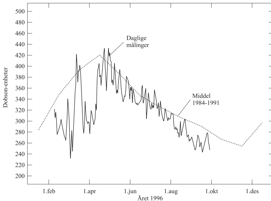
Figur 2: Daglige ozonverdier målt med Dobson- og Brewer-instrumentene ved Universitetet i Tromsø i 1996. Den stiplede kurven er månedsmidlene fra 1984 til 1991.
