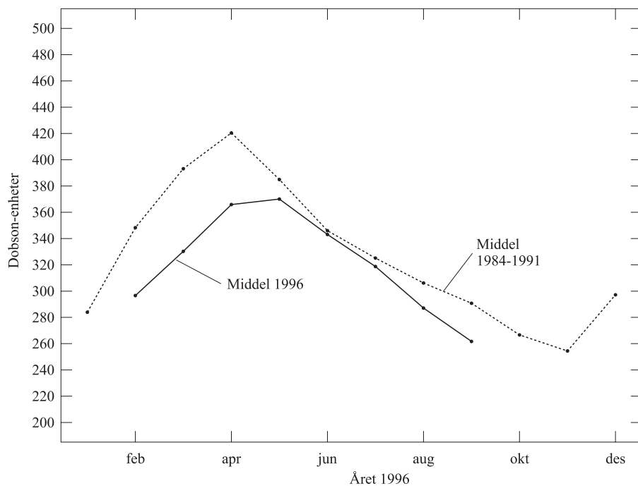
Figur 5: Månedsmiddelverdiene for 1996 og månedsmiddelverdiene for 1984 til 1991 for Tromsø.
