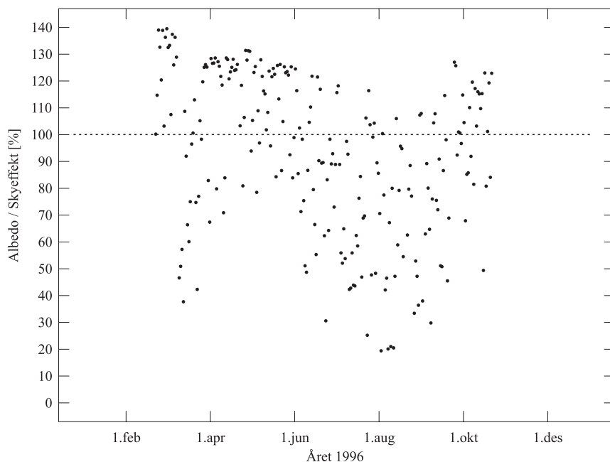
Figur 28: Effekter av skyer og bakkealbedo på UV-stråling ved jordens overflate i Ny-Ålesund i 1996 i prosent av klarværsverdien med null bakkerefleksjon. Hvert punkt representerer middelverdien mellom 10:30 og 11:30 GMT for en bestemt dag. Den horisontale linjen representerer klarvær og barmark. Verdier over denne linjen betyr at skyer og/eller bakkealbedo øker UV-nivået sammenlignet med klarvær og bar bakke.
