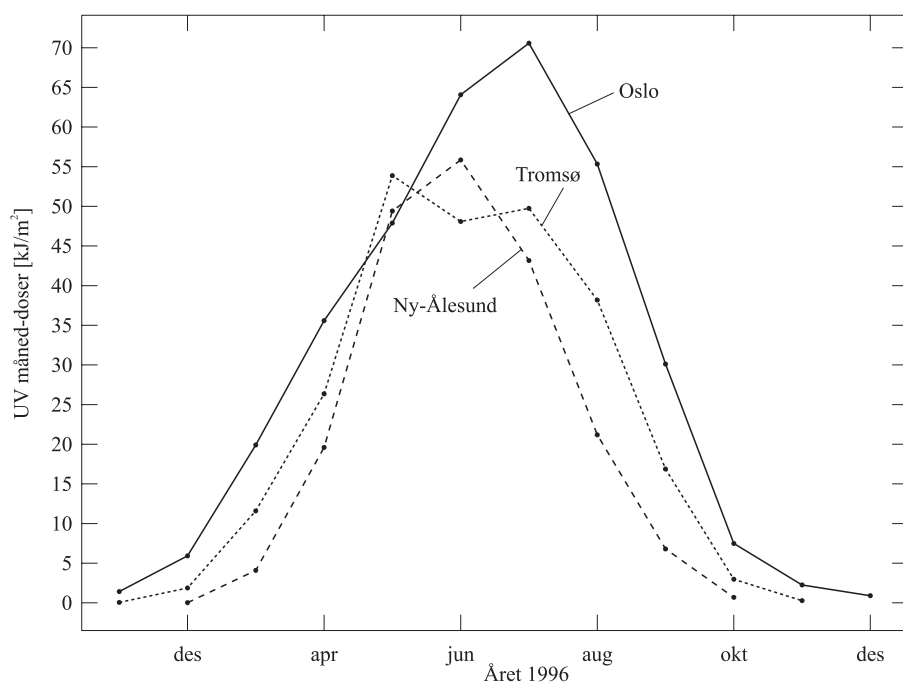
Figur 24: Månedlige integrerte UV-doser i 1996 målt med GUV-instrumentene i Oslo, Tromsø og Ny-Ålesund.
