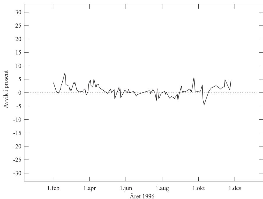
Figur 17: Sammenligning mellom ozonmålinger utført med Dobson og GUV-511 for Oslo in 1996, 100 \cdot (\text{Dobson-GUV}) / \text{Dobson} .
