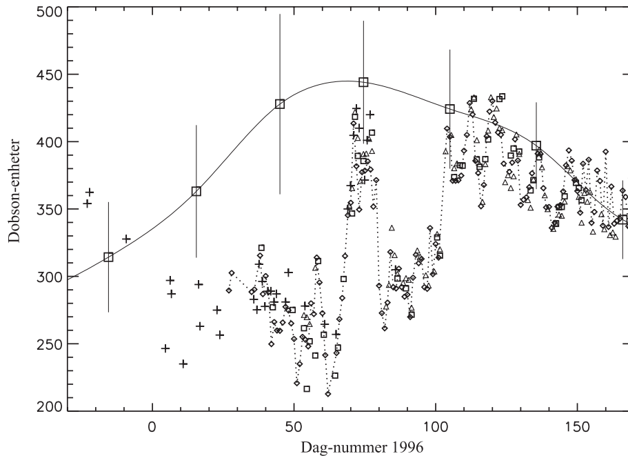
Figur 12: Målinger av totalozon fra Andøya (lidar) og Tromsø (Dobson, GUV og Brewer). Lidar målingene er markert med +. Langtidsmålinger med Dobson-instrumentet i Tromsø i perioden 1950-1972 er foreløpige data.
