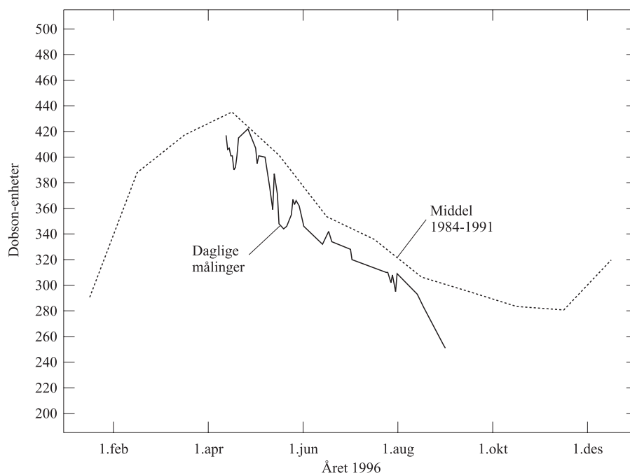
Figur 3: Daglige ozonverdier målt med Dobson-instrumentet i Ny-Ålesund 1996. Den stiplete kurven er månedsmidler fra 1984 til 1991.
