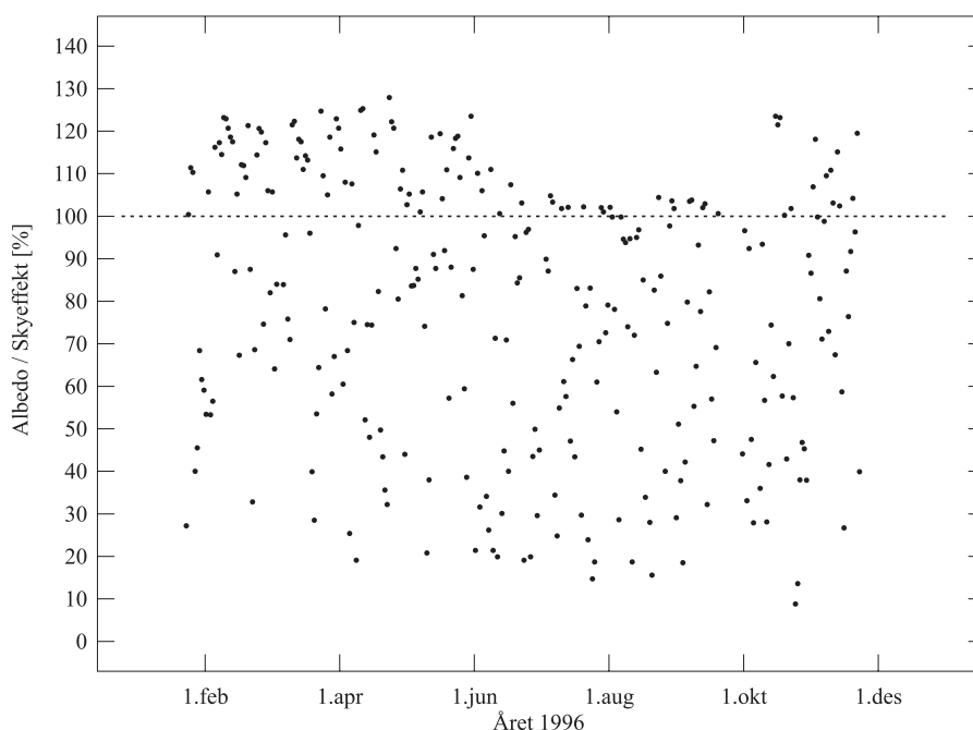
Figur 27: Effekter av skyer og bakkealbedo på UV-stråling ved jordens overflate i Tromsø i 1996 i prosent av klarværsverdien med null bakkerefleksjon. Hvert punkt representerer middelveidien mellom 10:30 og 11:30 GMT for en bestemt dag. Den horisontale linjen representerer klarvær og barmark. Verdier over denne linjen betyr at skyer og/eller bakkealbedo øker UV-nivået sammenlignet med klarvær og bar bakke.
