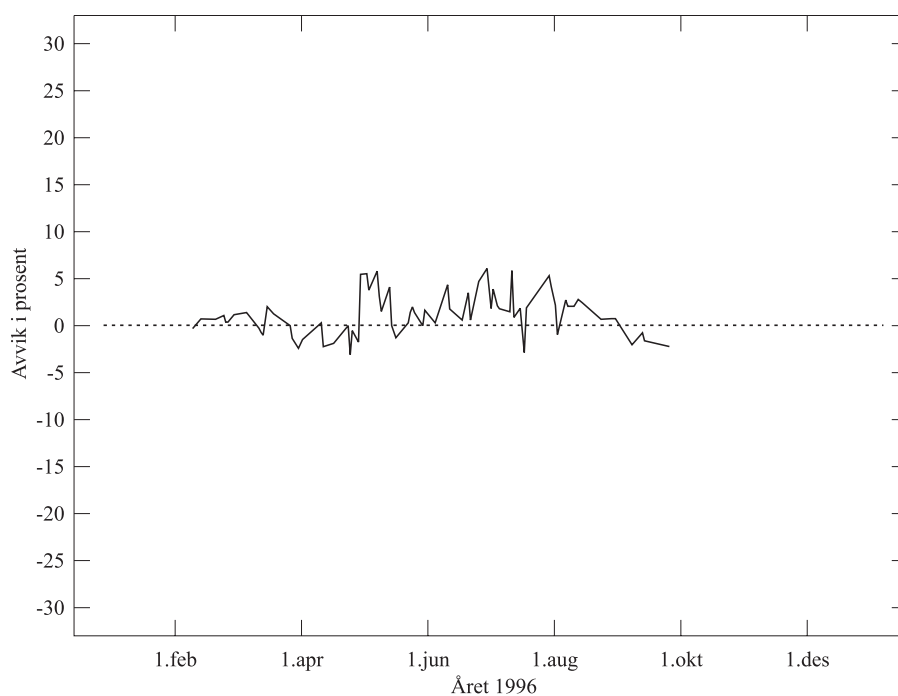
Figur 18: Sammenligning mellom ozonmålinger utført med Dobson- og Brewer-instrumentet for Tromsø i 1996, 100 \cdot (Dobson - Brewer) / Dobson .
