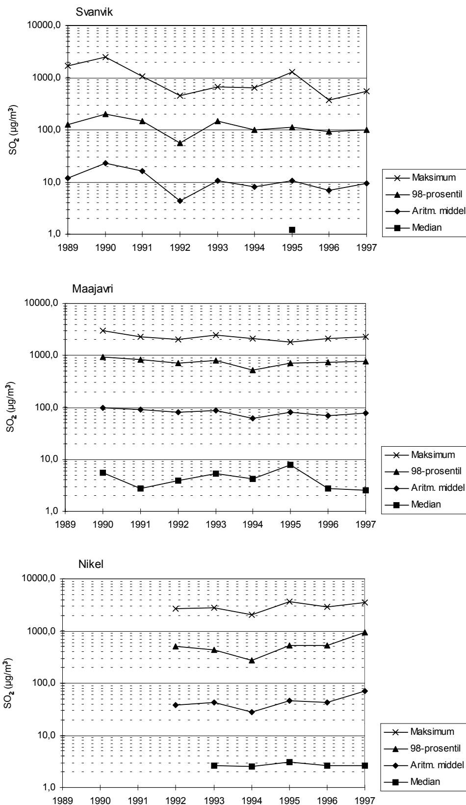
Figur 7: Timemiddelkonsentrasjoner av \text{SO}_2 i vinterhalvåret (oktober-mars) i Svanvik, Maajavri og Nikel ( \mu\text{g}/\text{m}^3 ). Trend for utvalgte statistiske parametre.
