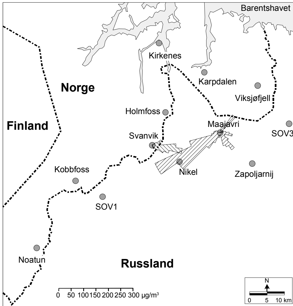
Figur 3: Middelkonsentrasjoner av \text{SO}_2 for Svanvik og Maajavri i 36 vindsektorer i perioden oktober 1996-mars 1997 ( \mu\text{g}/\text{m}^3 ).
