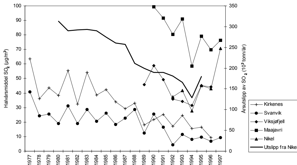
Figur 5: Vintermiddelskonsentrasjoner (oktober-mars) av SO_2 i perioden 1977-1997 ( \mu\text{g}/\text{m}^3 ). Figuren viser også årlige utslipp av SO_2 fra smelteverket i Nikel i perioden 1980-1995 ( 10^3 tonn/år).
