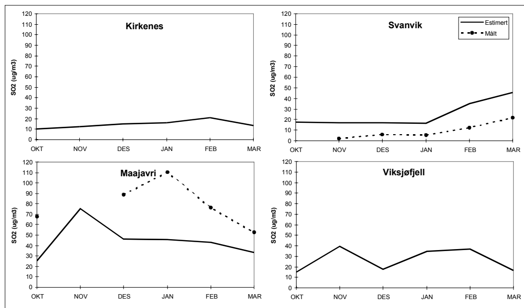
Figur 11: Målte og beregnede månedsmiddelkonsentrasjoner (oktober 1996-mars 1997) av svoveldioksid på de respektive stasjonene (µg/m³).
