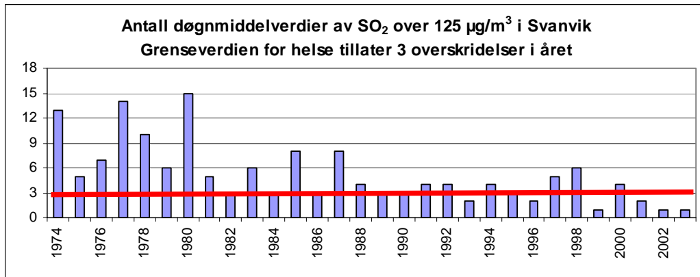
Figur 9: Antall døgnmiddelverdier av SO 2 over grenseverdien på 125 µg/m 3 i Svanvik i årene 1974-2003 (3 tillatte overskridelser i året).
