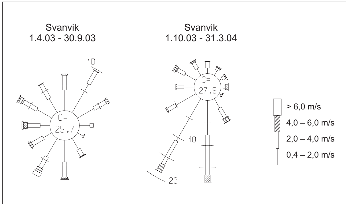
Figur 2: Vindrosen fra Svanvik for periodene april-september 2003 og oktober 2003-mars 2004. (Vindrosene viser frekvensen av vind i tolv 30-graders sektorer, dvs. hvor ofte det blåser fra disse retningene).
