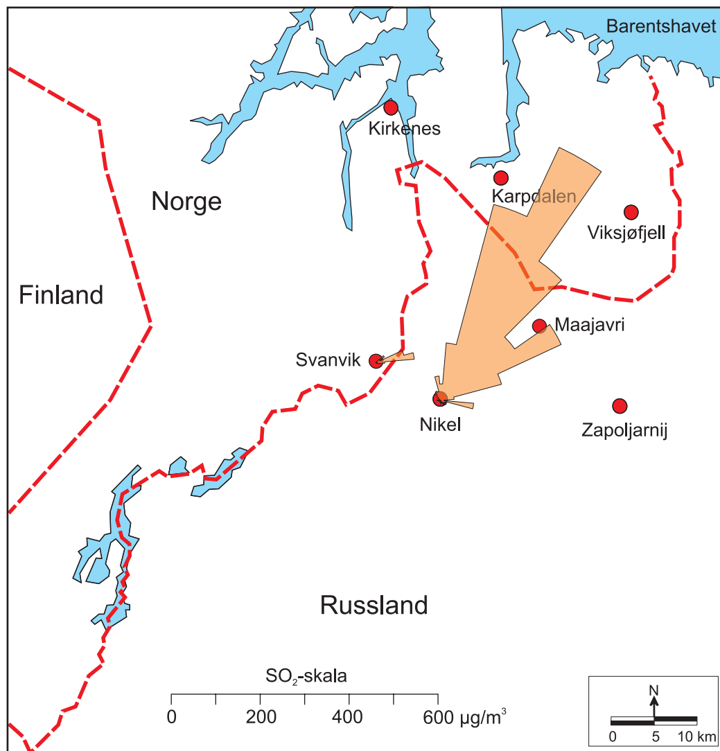
Figur 4: Middelskonsentrasjoner av SO 2 i Svanvik og Nikel i perioden oktober 2005-mars 2006 (µg/m 3 ). Figuren viser middelskonsentrasjoner av SO 2 for hver av 36 10°-vindsektorer. Svanvik er belastet fra Nikel og Zapoljarnij (mest fra Nikel).
