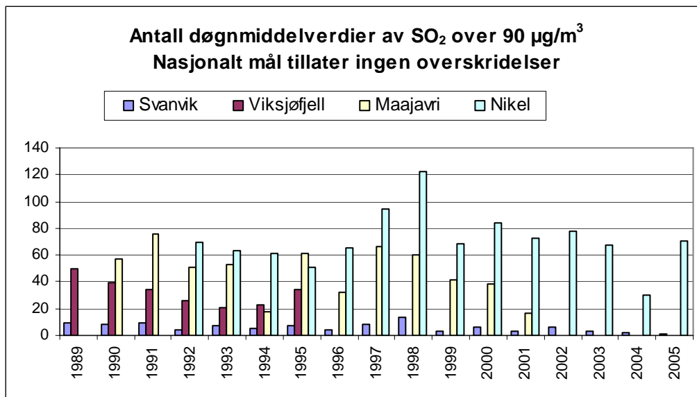
Figur 13: Antall døgnmiddelverdier av SO 2 over Nasjonalt mål på 90 µg/m 3 i Svanvik (1989-2005), på Viksjøfjell (1989-1995), i Maajavri (1990-2001) og i Nikel (1992-2005) (ingen tillatte overskridelser).
