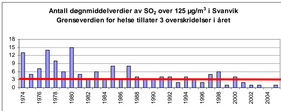
Figur 9: Antall døgnmiddelverdier av SO 2 over grenseverdien på 125 µg/m 3 i Svanvik i årene 1974-2005 (3 tillatte overskridelser i året).
