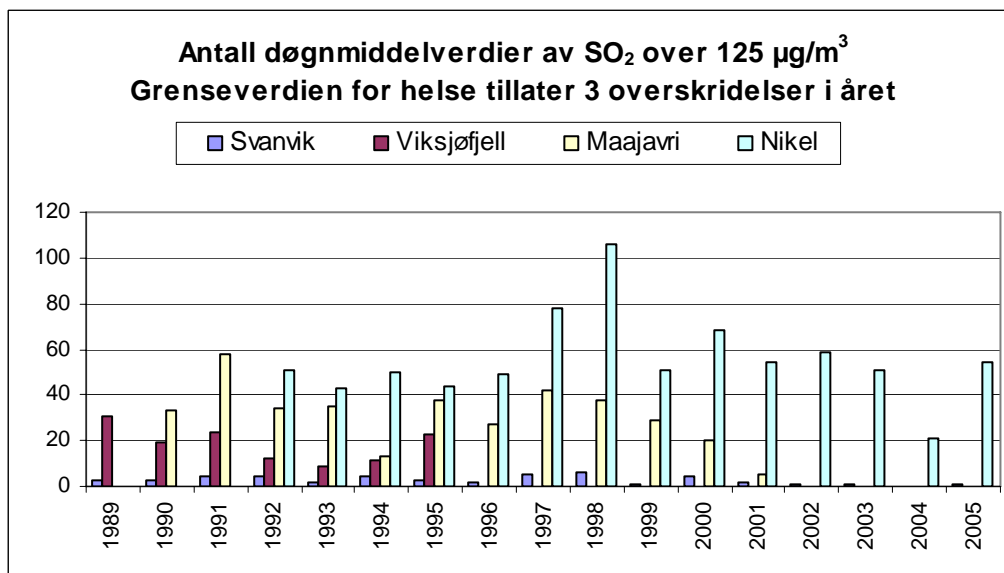
Figur 10: Antall døgnmiddelverdier av SO 2 over grenseverdien på 125 µg/m 3 i Svanvik (1989-2005), på Viksjøfjell (1989-1995), i Maajavri (1990-2001) og i Nikel (1992-2005) (3 tillatte overskridelser i året).
