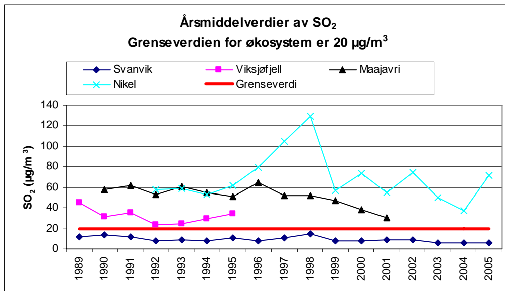
Figur 6: Årsmiddelverdier av SO 2 i Svanvik (1989-2005), på Viksjøfjell (1989-1995), i Maajavri (1990-2001) og i Nikel (1992-2005) (µg/m 3 ).
