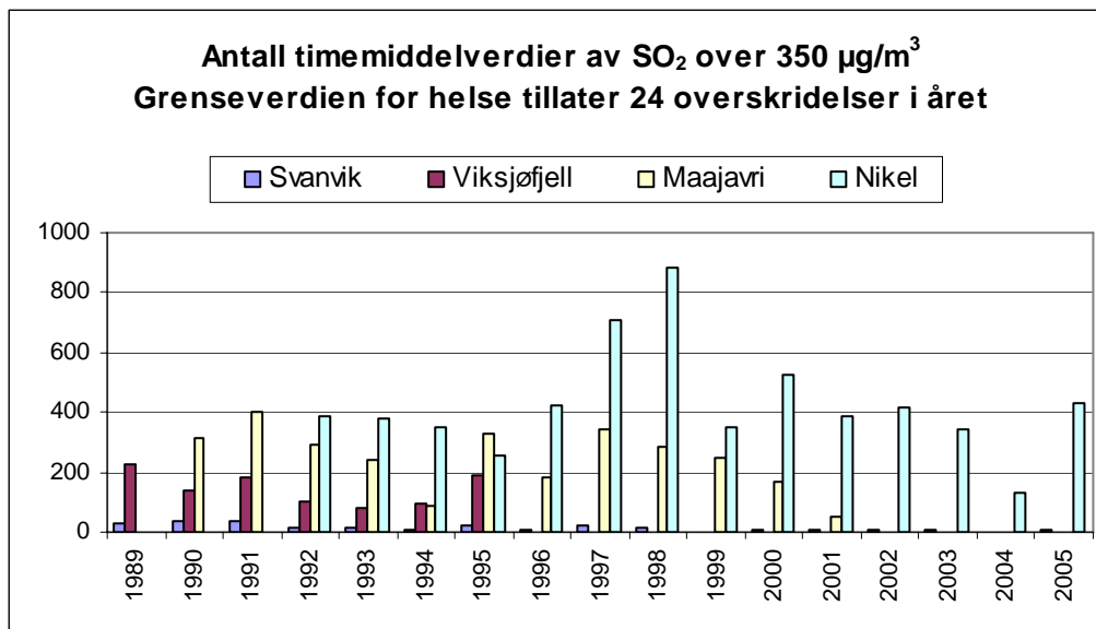
Figur 15: Antall timemiddelverdier av SO 2 over grenseverdien på 350 µg/m 3 i Svanvik (1989-2005), på Viksjøfjell (1989-1995), i Maajavri (1990-2001) og i Nikel (1992-2005) (24 tillatte overskridelser i året).
