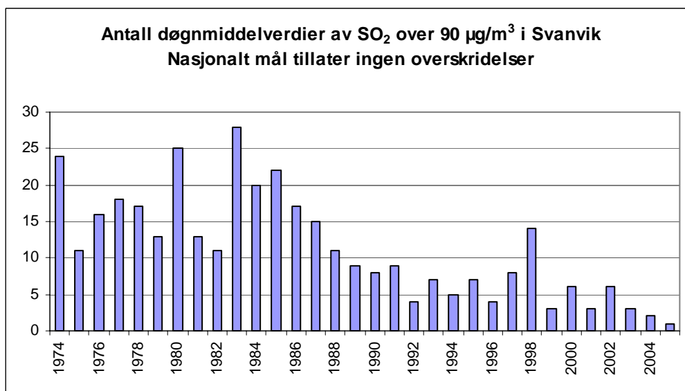
Figur 12: Antall døgnmiddelverdier av SO_2 over Nasjonalt mål på 90 \mu g/m^3 i Svanvik i årene 1974-2005 (ingen tillatte overskridelser).
