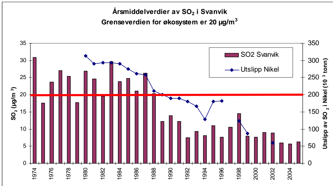
Figur 5: Årsmiddelverdier av SO 2 i Svanvik i årene 1974-2005 (µg/m 3 ).
