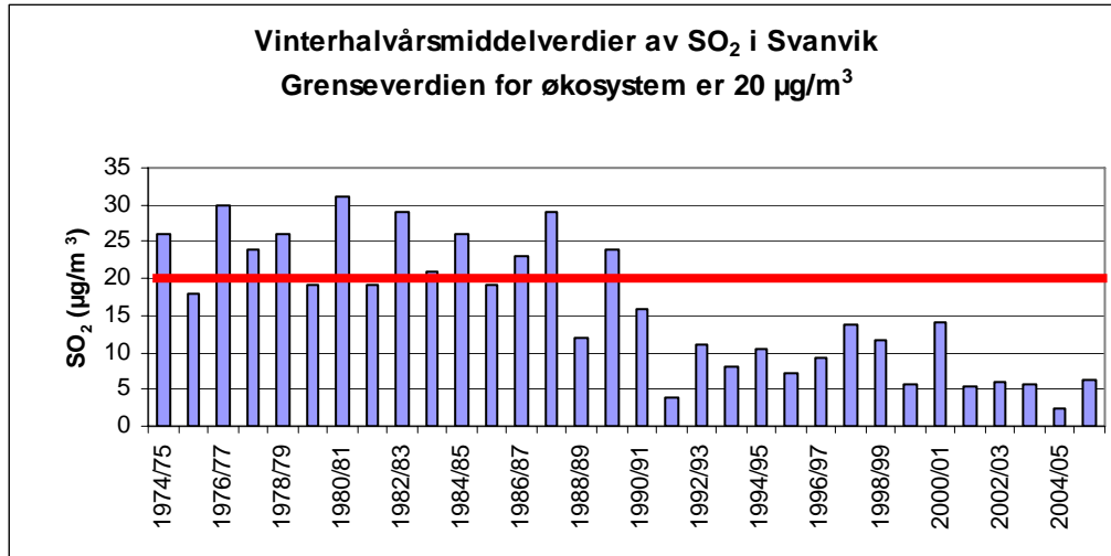
Figur 7: Vinterhalvårsmiddelverdier av SO 2 i Svanvik 1974/75-2005/06 (µg/m 3 ).
