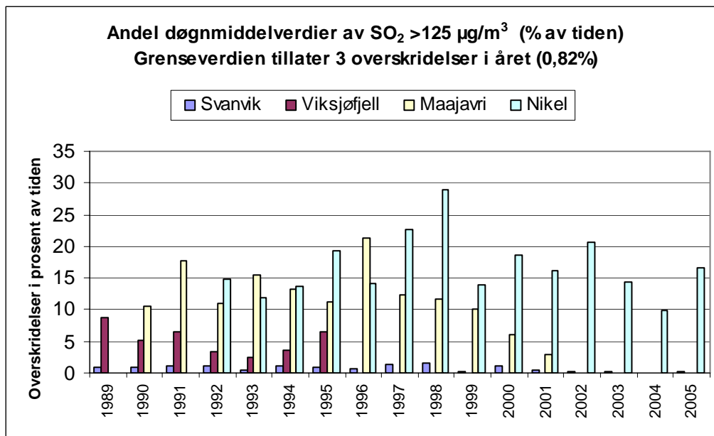
Figur 11: Andel av tiden grenseverdien for døgnmiddel av SO_2 på 125 \mu g/m^3 er overskredet i Svanvik (1989-2005), på Viksjøfjell (1989-1995), i Maajavri (1990-2001) og i Nikel (1992-2005) (3 tillatte overskridelser i året tilsvarer 0,82% av tiden).
