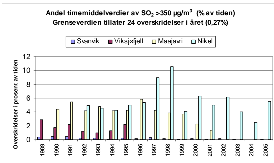
Figur 16: Andel av tiden grenseverdien for timemiddel av SO 2 på 350 µg/m 3 er overskredet i Svanvik (1989-2005), på Viksjøfjell (1989-1995), i Maajavri (1990-2001) og i Nikel (1992-2005) (24 tillatte overskridelser i året tilsvarer 0,27% av tiden).
