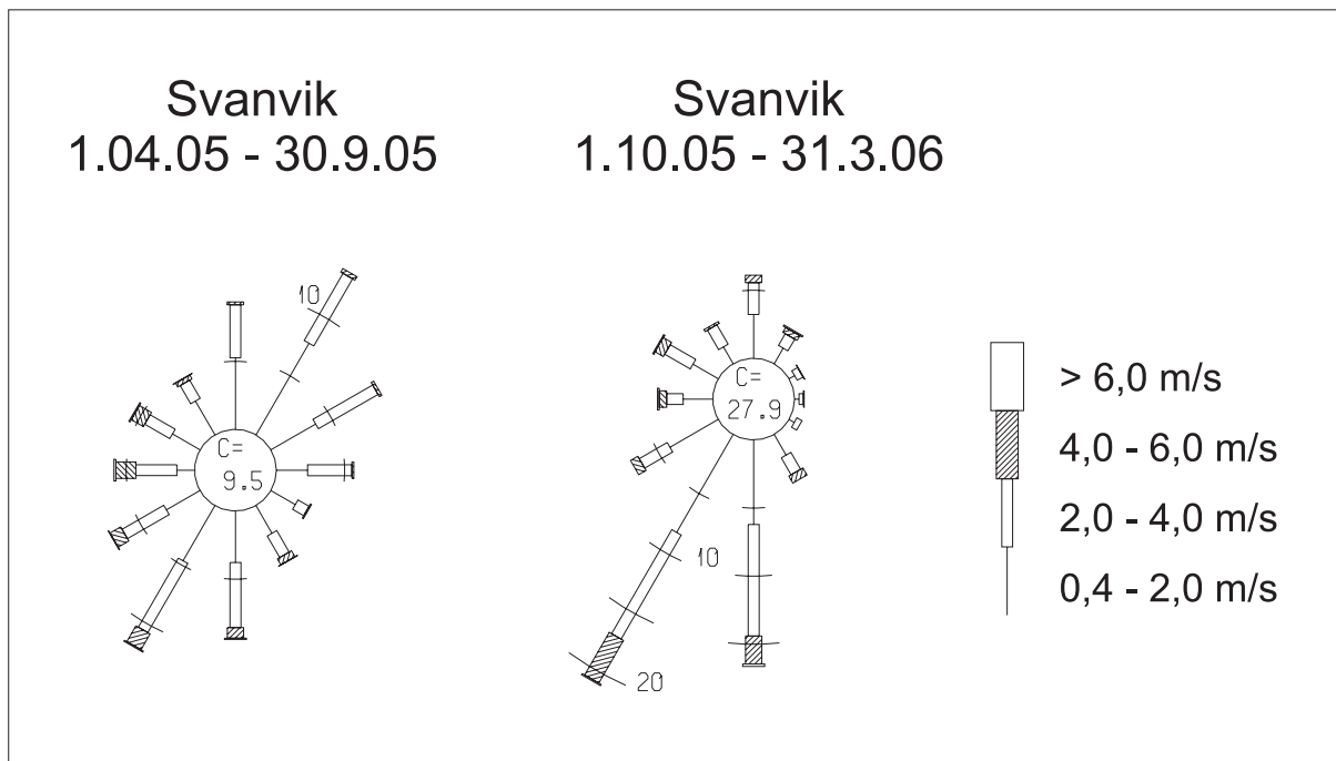
Figur 2: Vindrosen fra Svanvik for periodene april-september 2005 og oktober 2005-mars 2006. (Vindrosene viser frekvensen av vind i tolv 30-graders sektorer, dvs. hvor ofte det blåser fra disse retningene).
