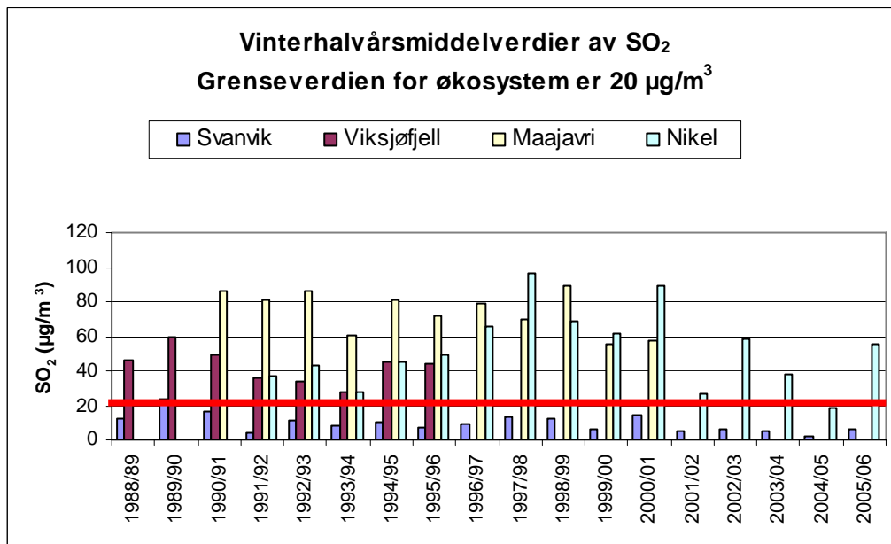
Figur 8: Vinterhalvårsmiddelverdier av SO 2 i Svanvik (1988/89-2005/06), på Viksjøfjell (1988/89-1995/96), i Maajavri (1990/91-2000/01) og i Nikel (1991/92-2005/06) (µg/m 3 ).
