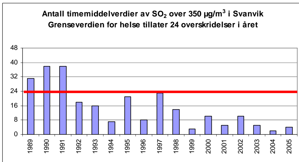
Figur 14: Antall timemiddelverdier av SO 2 over grenseverdien på 350 µg/m 3 i Svanvik i årene 1989-2005 (24 tillatte overskridelser i året).
