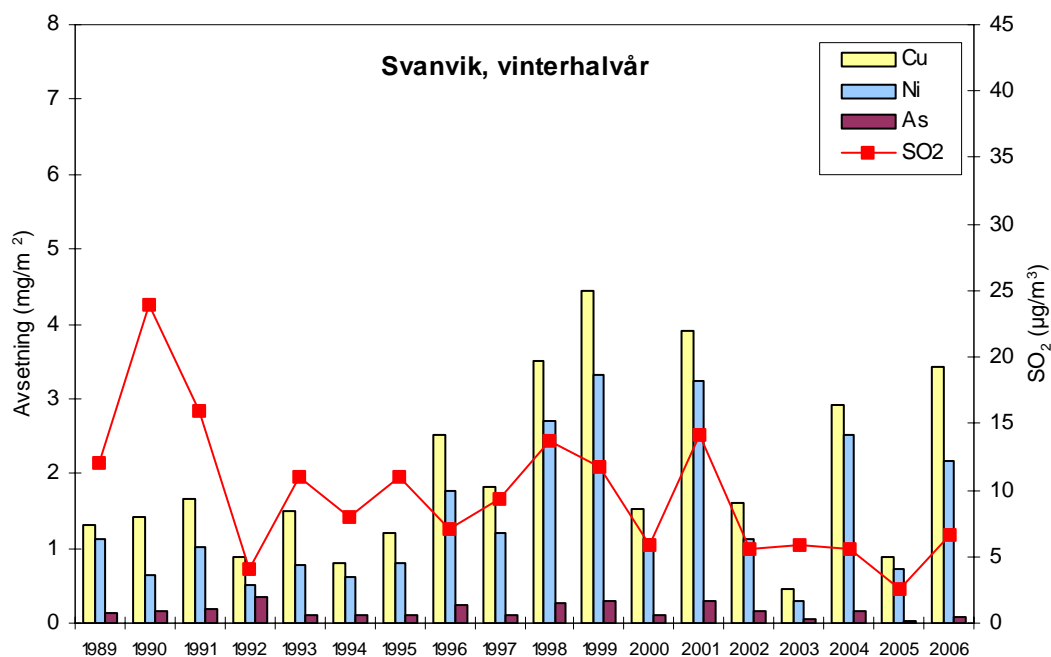
Figur 17: Avsetning med nedbør av Cu, Ni og As (mg/m 2 ) i sommerhalvårene fra 1989 til 2005 og i vinterhalvårene fra 1988/89 til 2005/06. Halvårsmiddelkonsentrasjonene av SO 2 er også vist (µg/m 3 ).
